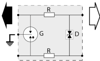
Р: 3-электродный GDT R: резистор D: фиксирующий диод
