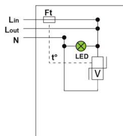
V: Варистор Ft: тепловой предохранитель LED: индикатор отключения t°: Система термического отключения
