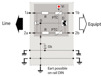
G: 3-электродная газовая трубка Gb: 2-электродная газовая трубка PTC: Терморезистор D: фиксирующий диод Vi: индикатор
